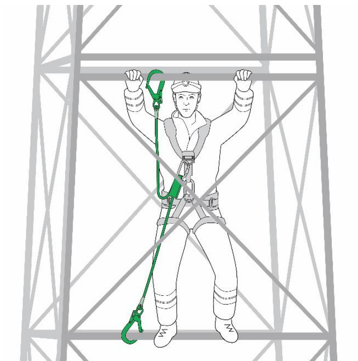
Rycina 9 – Wspinaczka po konstrukcji z lonżami z absorberem energii.
