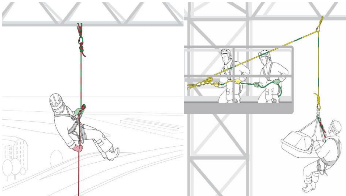
Rycina 12 - po lewej: zjazd w przrządzie z autoblokadą w technice jednej liny; - po prawej opuszczanie w technice jednej liny.
